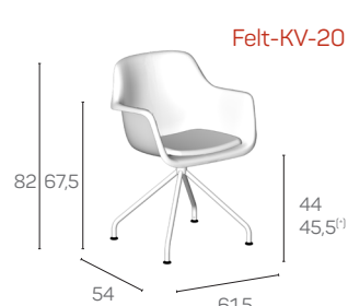
Felt-KV-20 kuip geperst vilt kruisvoet vast
