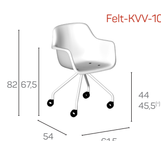
Felt-KVV-10 kuip geperst vilt kruisvoet met wielen
